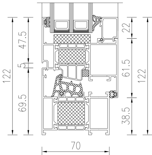
OKNO ALUPROF MB-79N SI
